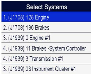
Scan ECU
